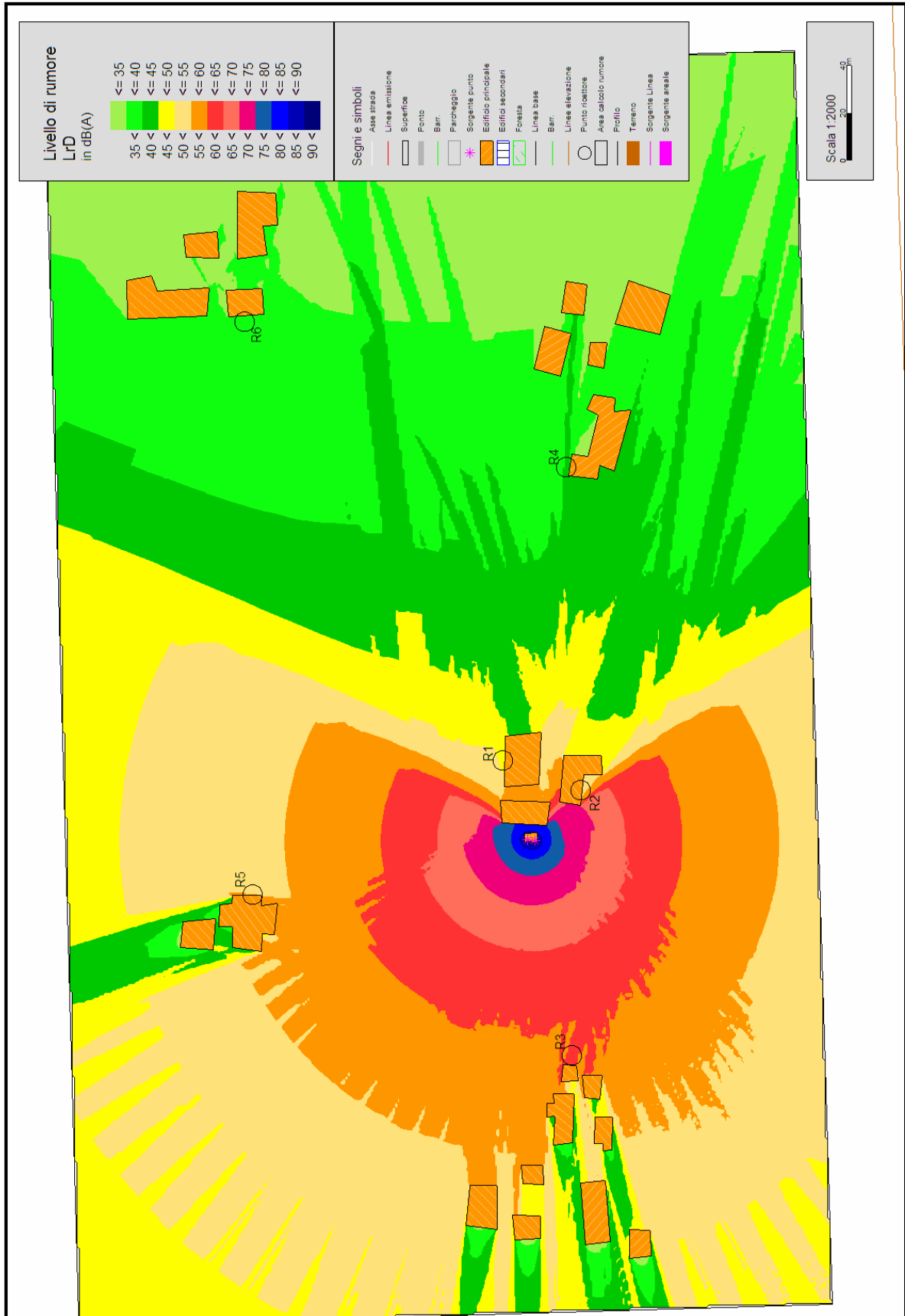
Fig. 3: Risultati della simulazione con SoundPlan 6.2 per l'impianto audio
