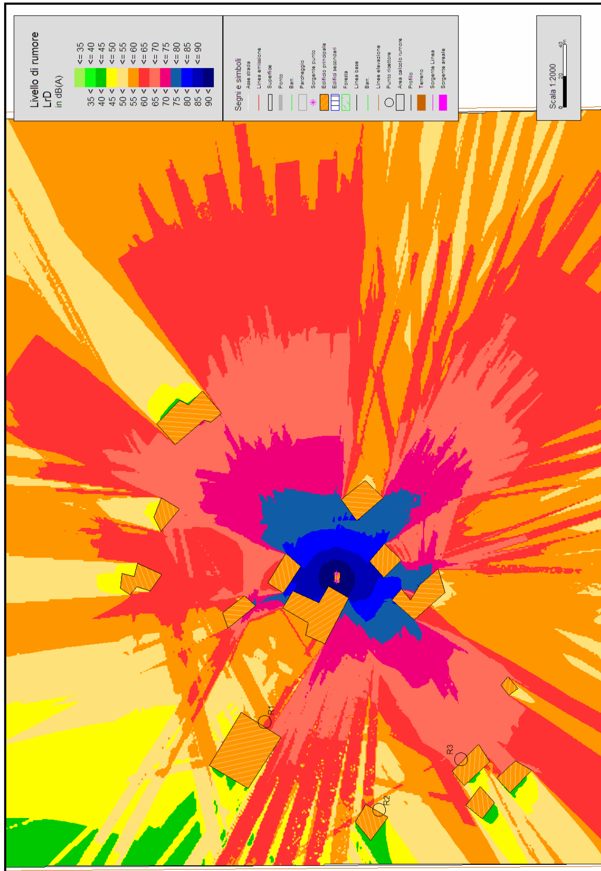
Fig. 3: Risultati della simulazione con SoundPlan 6.2 per l'impianto audio a 1,5 m di altezza
