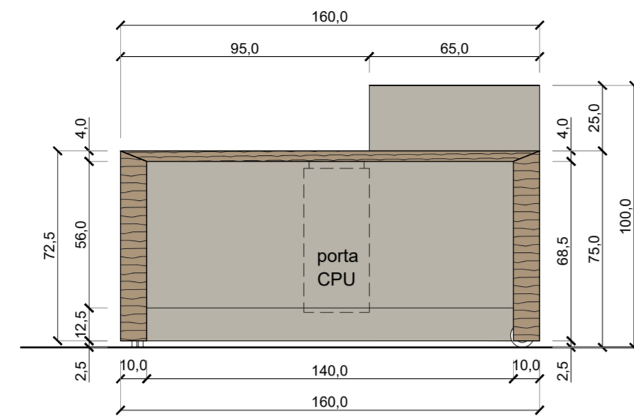
PROSPETTO RETRO
