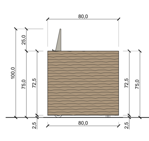
PROSPETTO LATERALE
