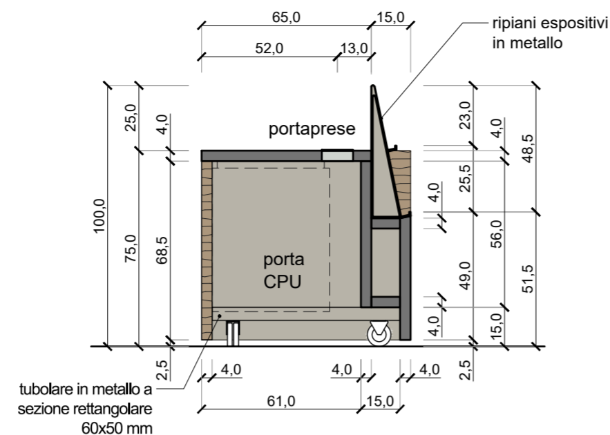
SEZIONE VERTICALE EE'
