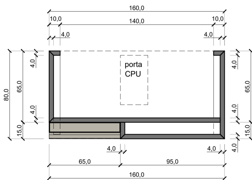
SEZIONE ORIZZONTALE AA'
