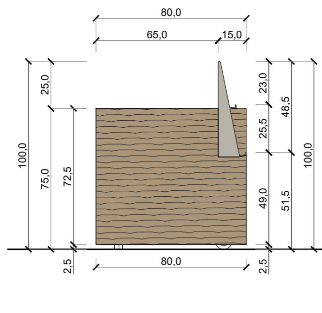
PROSPETTO LATERALE
