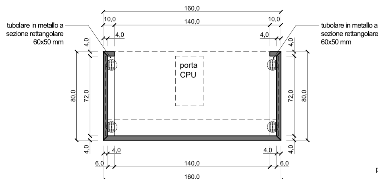
SEZIONE ORIZZONTALE CC'
