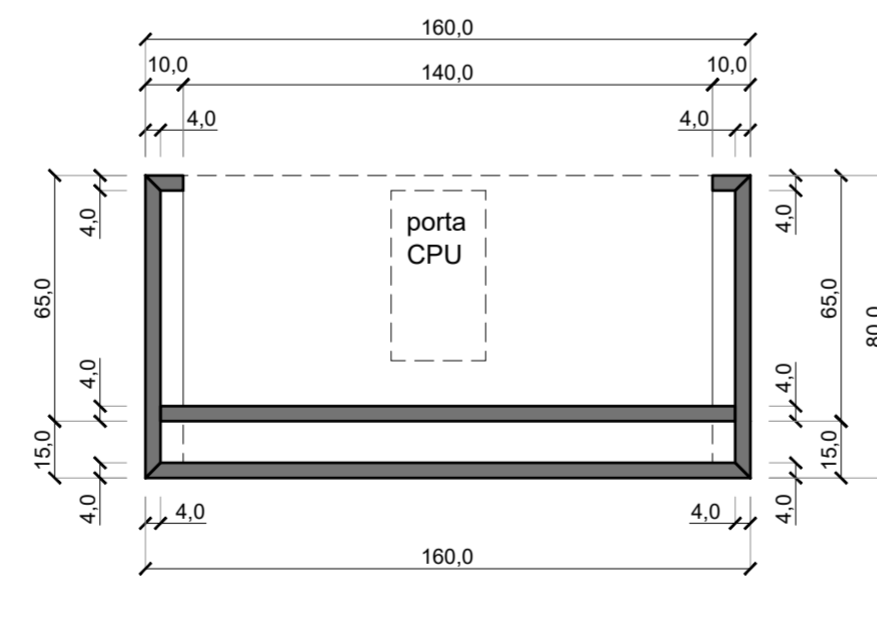
SEZIONE ORIZZONTALE BB'
