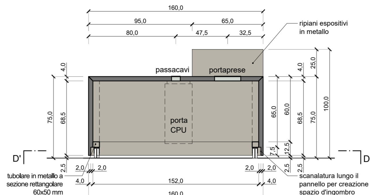
SEZIONE VERTICALE FF'
