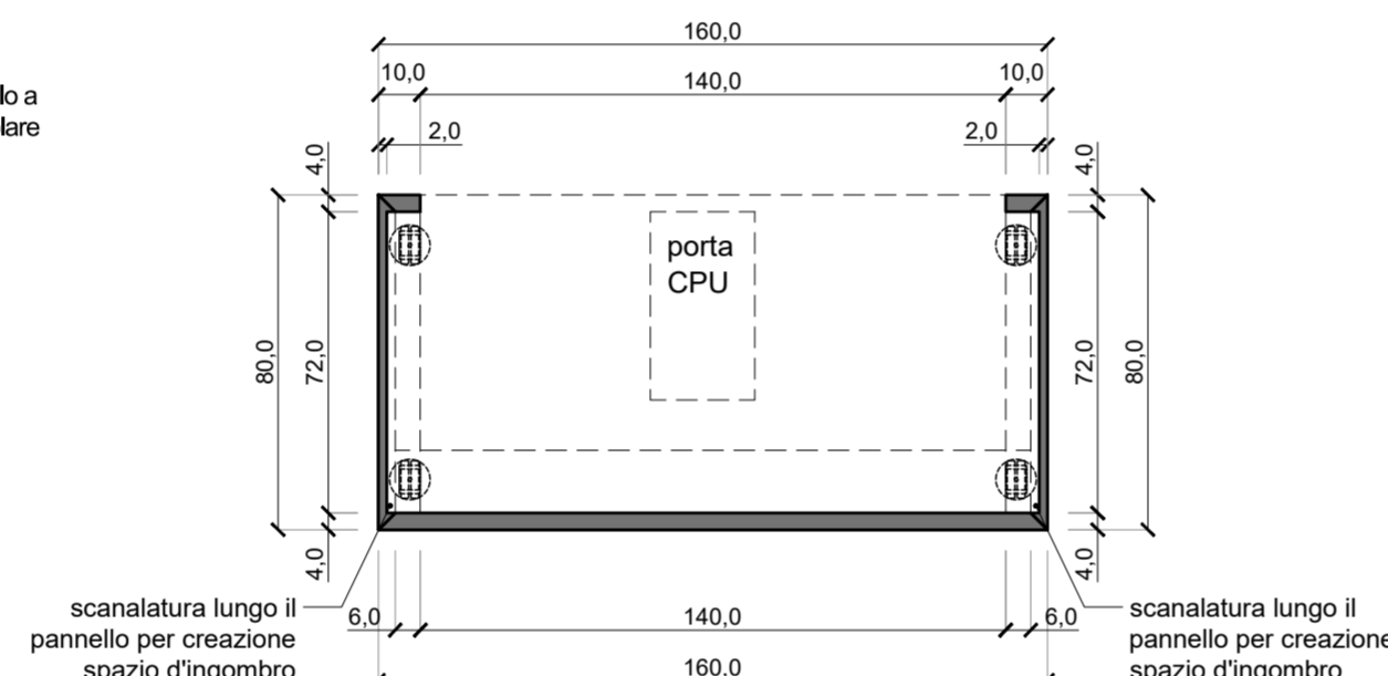
SEZIONE ORIZZONTALE DD'
