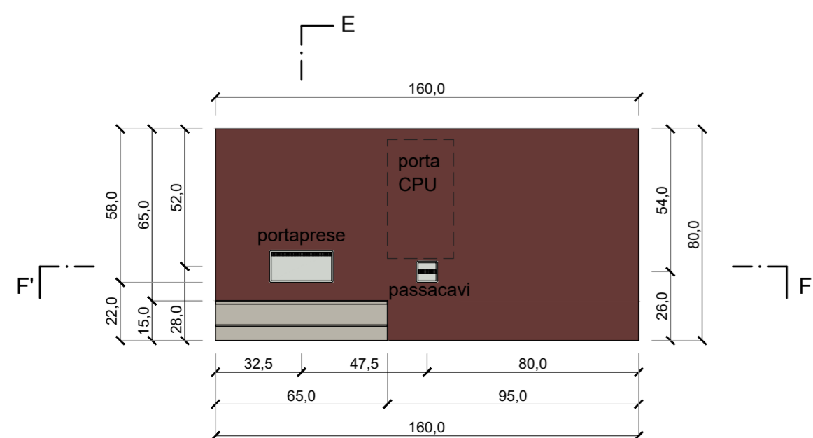
PIANTA cod. BA.04
