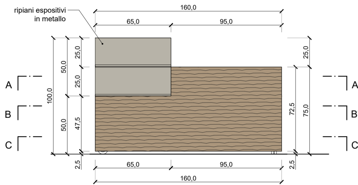
PROSPETTO FRONTALE
