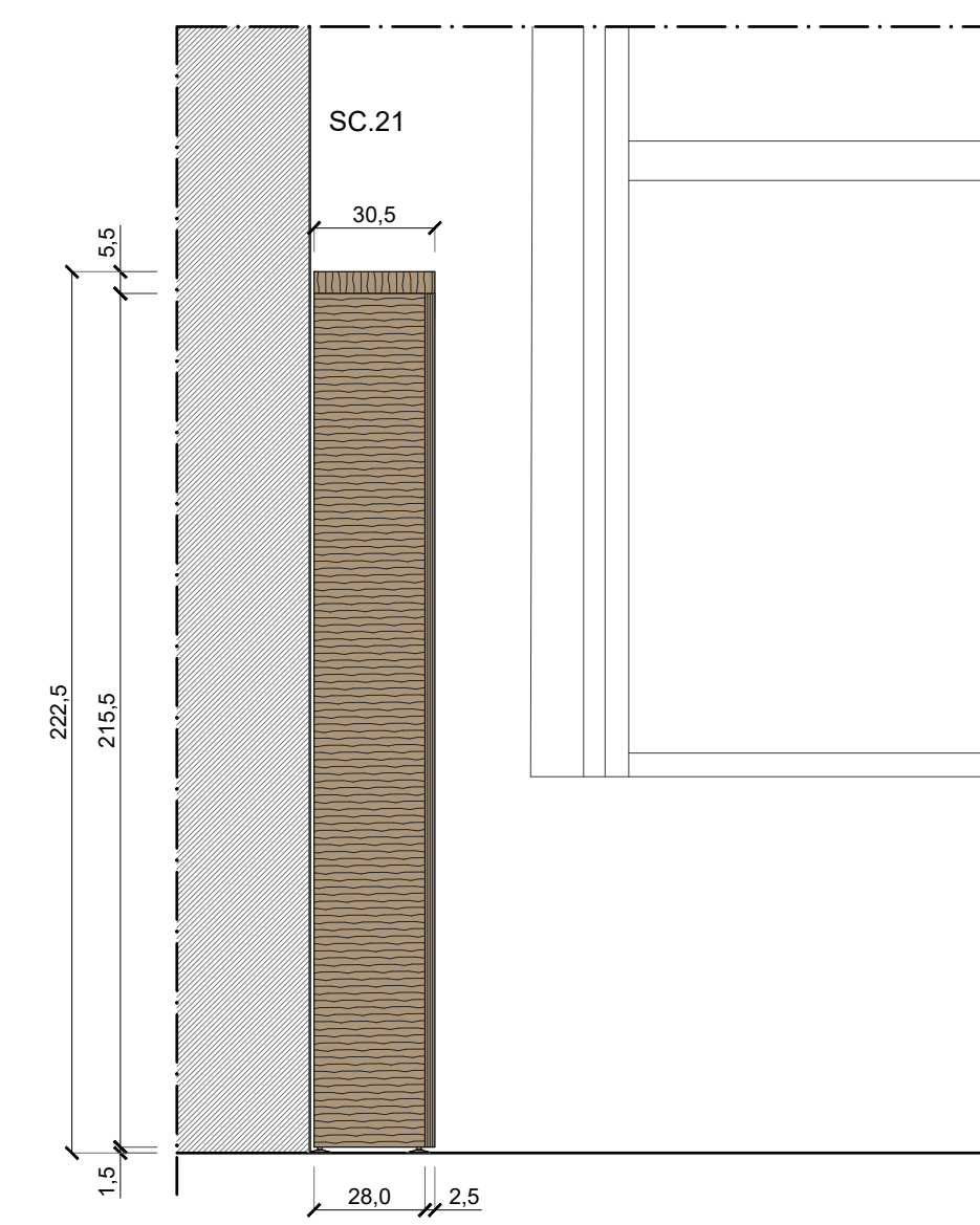
SEZIONE C-C'
