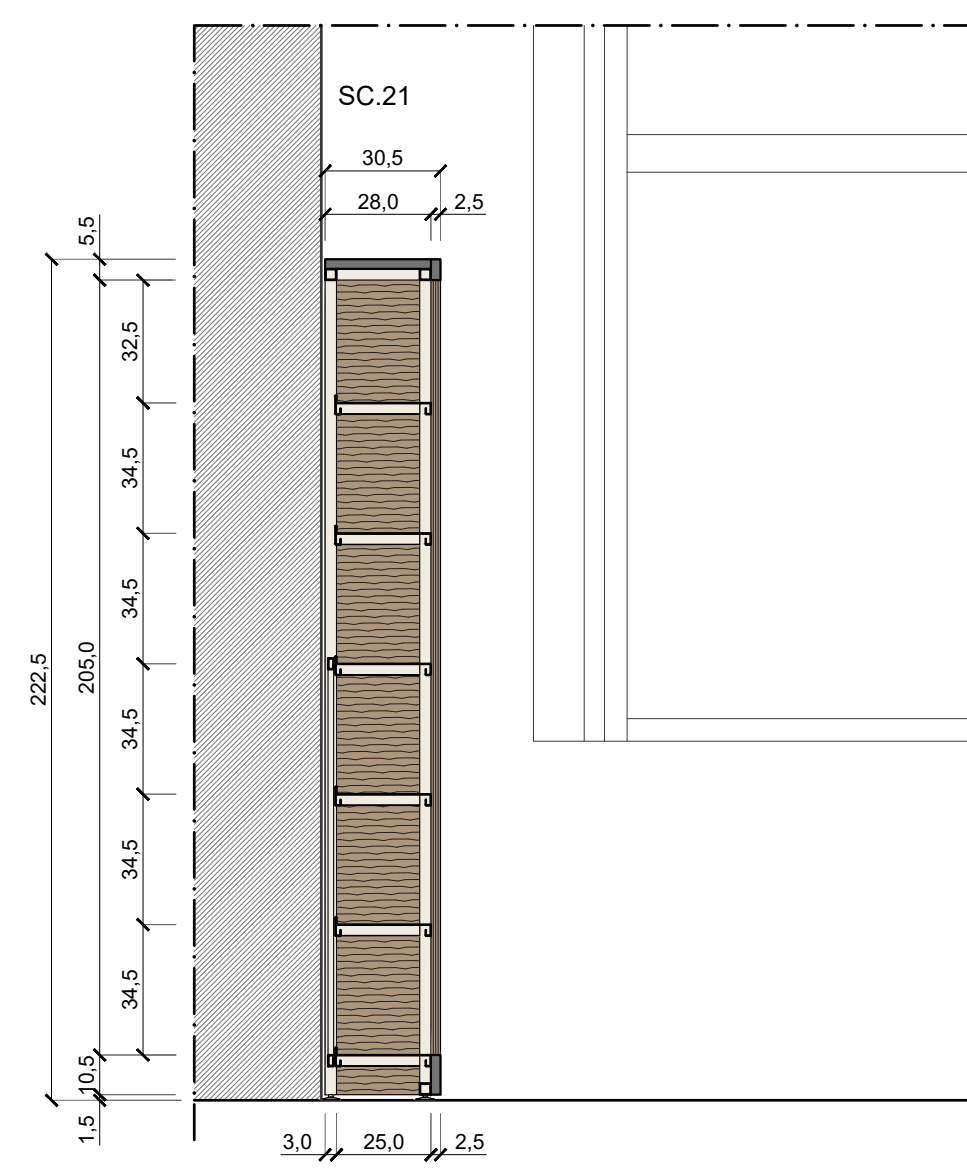
SEZIONE B-B'
