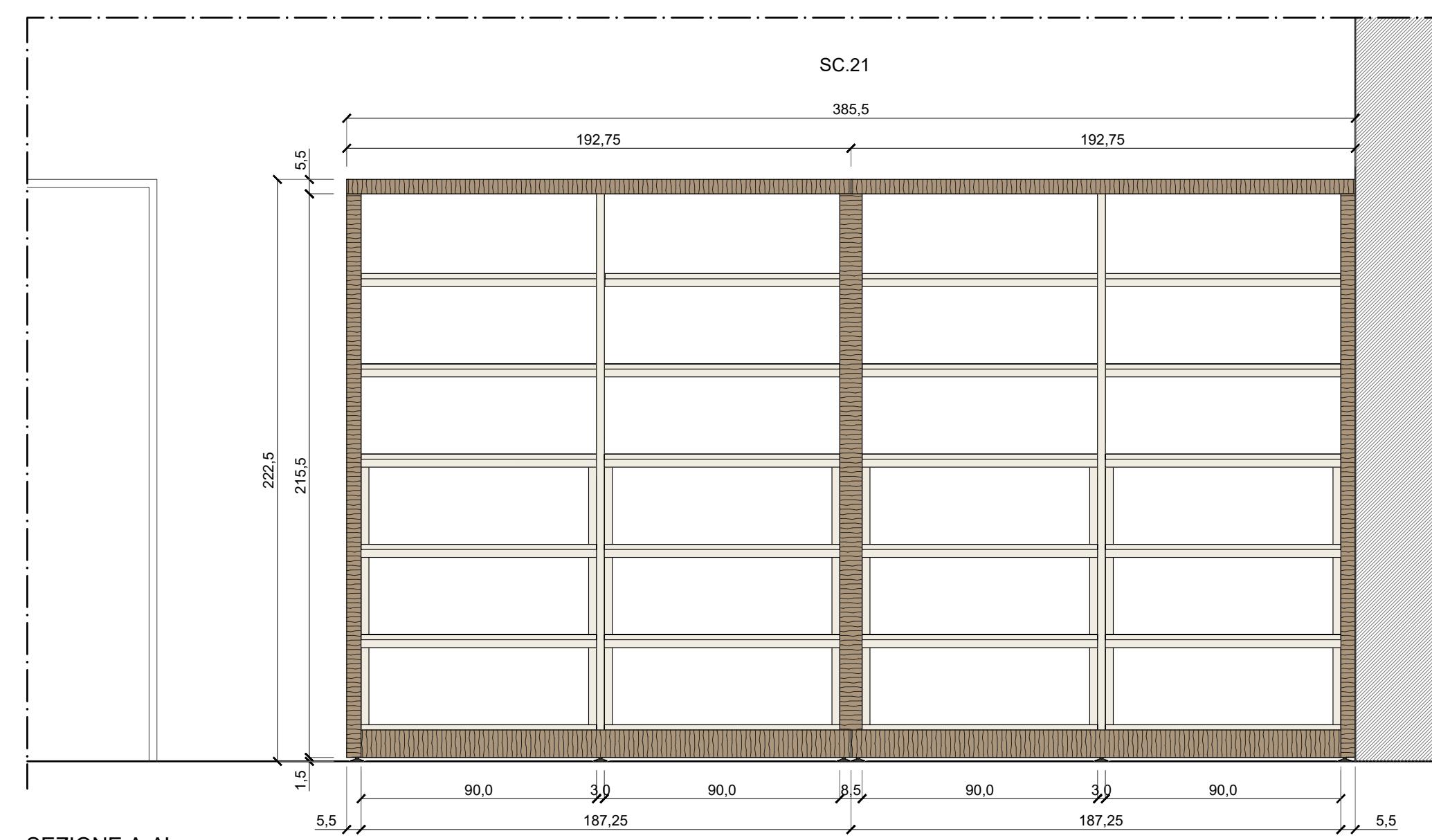
SEZIONE A-A'
