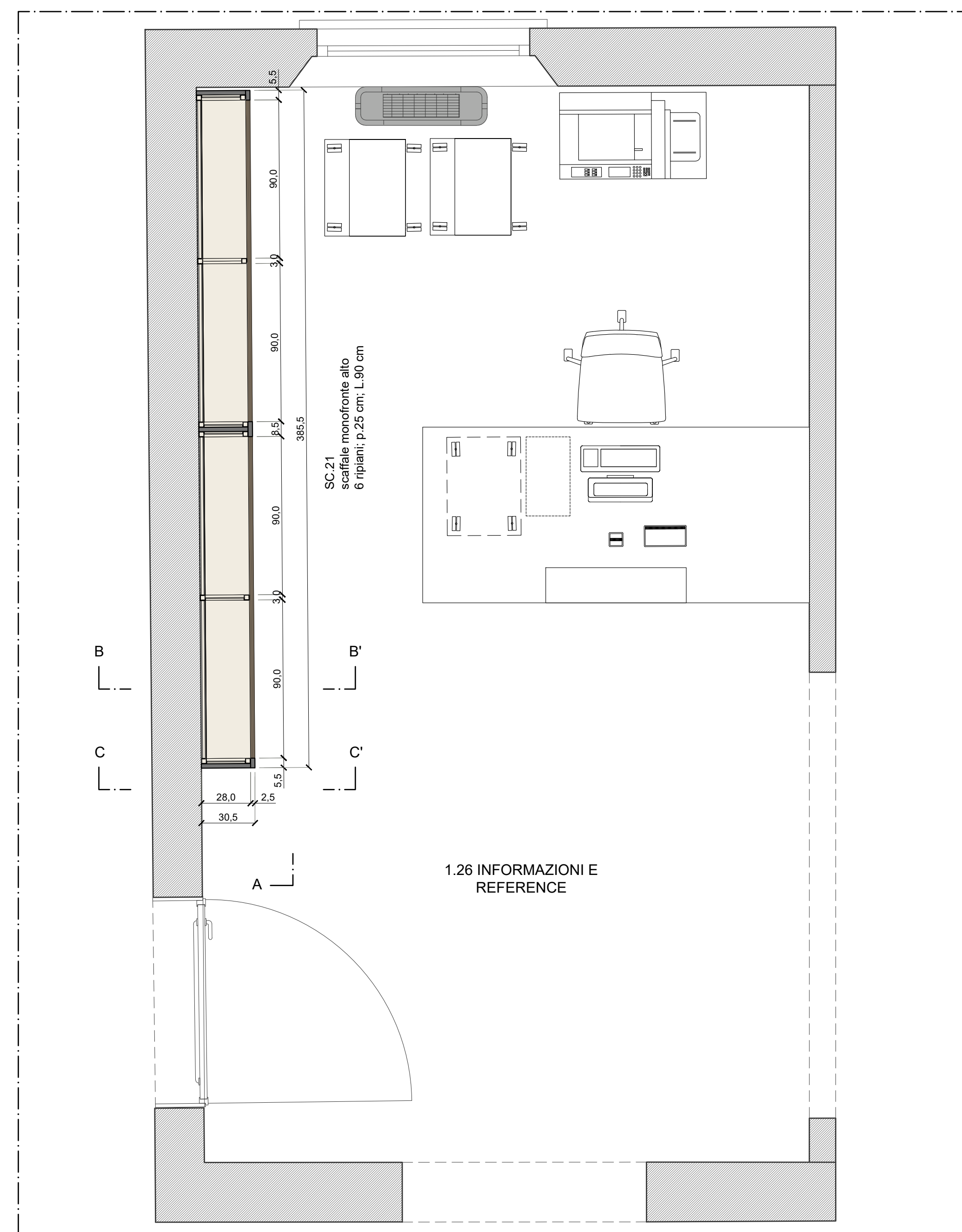
SEZIONE ORIZZONTALE
