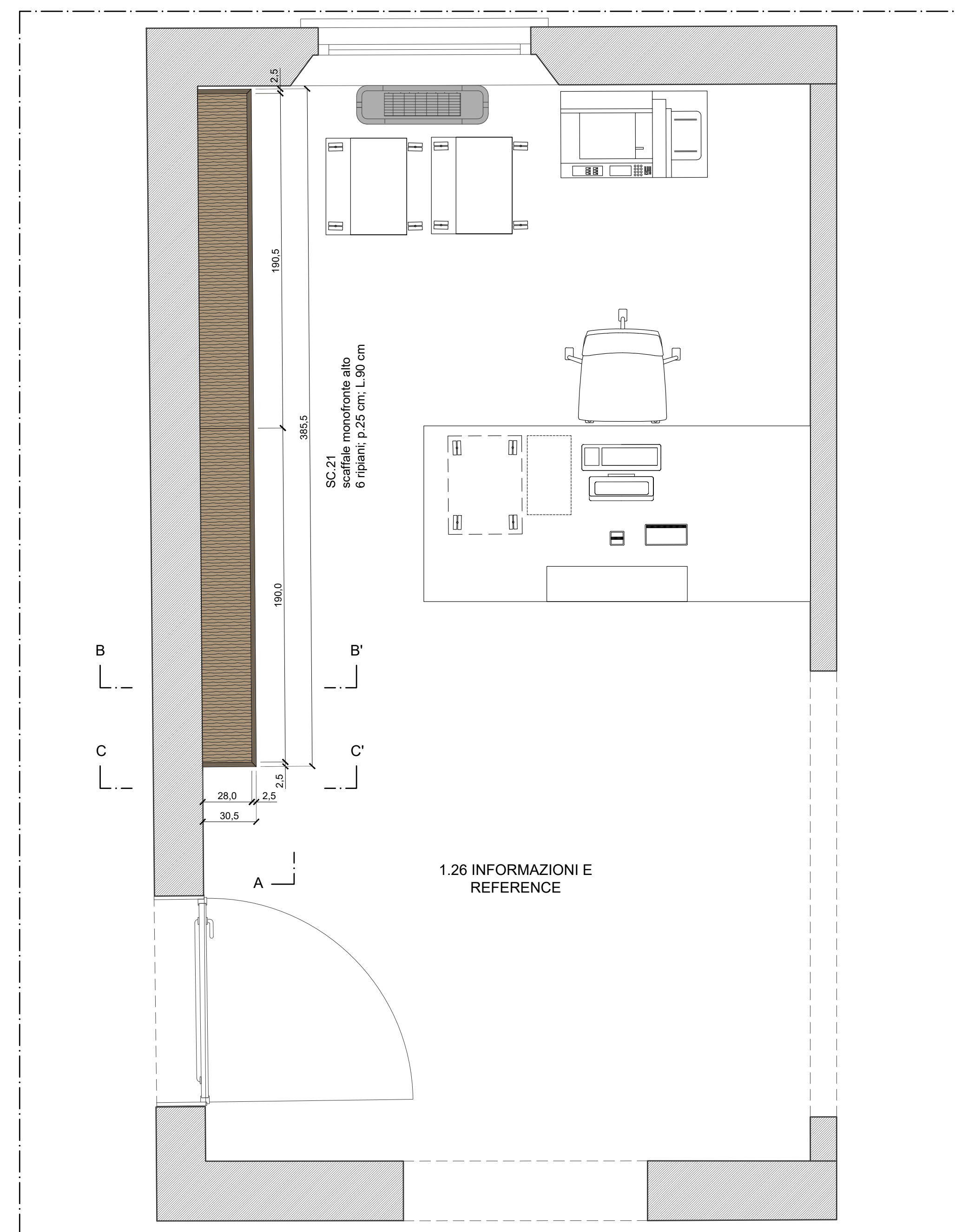
PIANTA (vista sopra il top)
